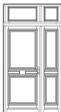
Imposte fixe, faux-ouvrant*
